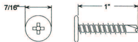
#12-14x1" Mini Point Pancake Head
