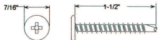
#14-13x1-1/2" Mini Point Pancake Head
