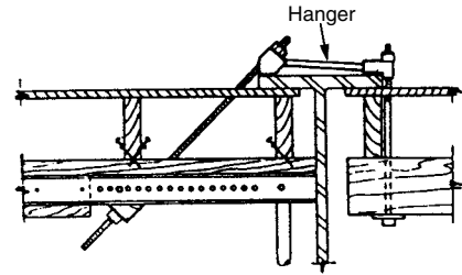
C-60 45° Pres-Steel Hanger, Type 4-A
