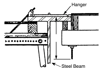
C-41 45° Coil Rod Hanger, Type 1-A
