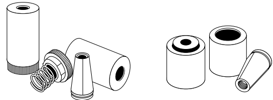
H-60-A CCL Spring Loaded Anchors
