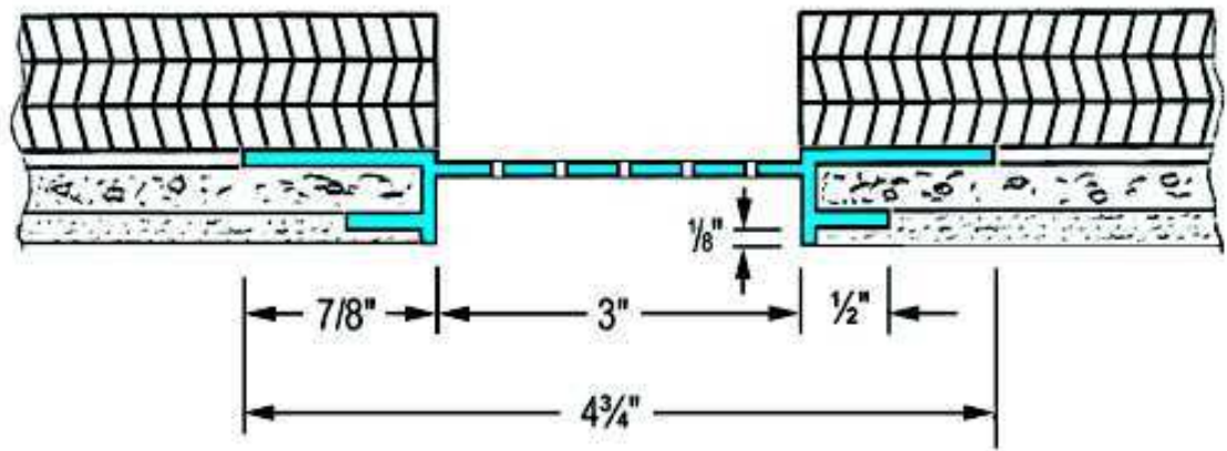
EIFS Soffit Vent
