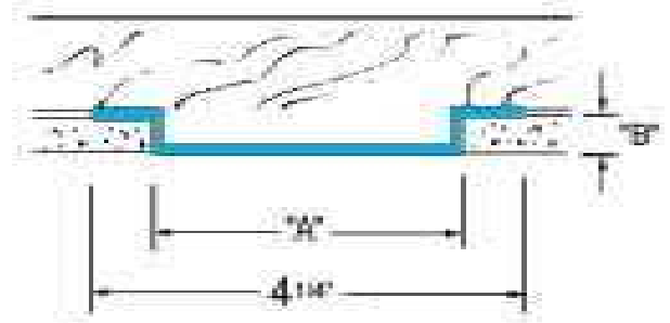
Drywall Soffit Vent Inserts
