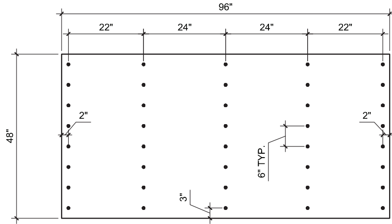
40 FASTENERS PER BD. (4'x8')
