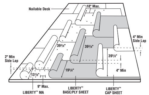
3-Ply Lay-out
