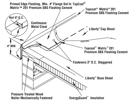
Edge Flashing
