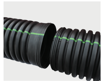
N-12 ST per AASHTO
