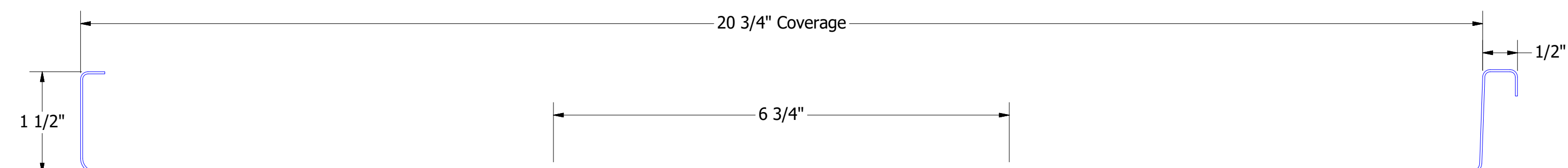
FLM207
