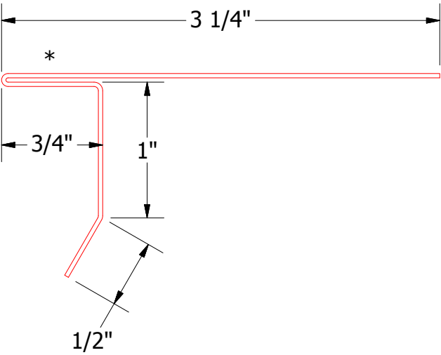
HSA114-Drip Edge
