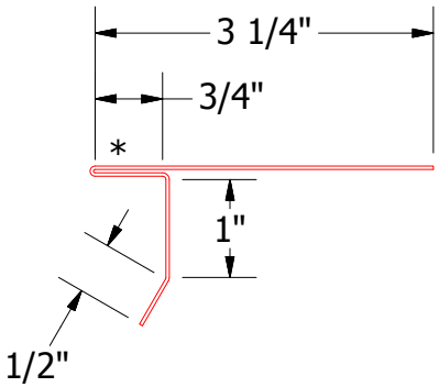
HSA114-Drip Edge
