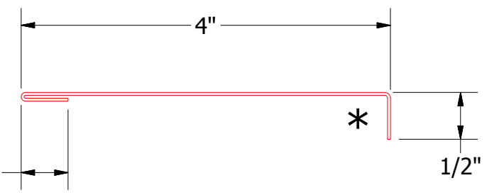
HCA671-Jamb Trim
