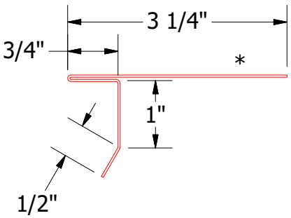
HLA112-Drip Edge
