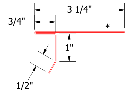
HLA112-Drip Edge
