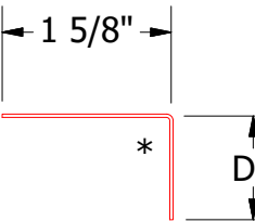
Angle Trim DWA680: D2= 1 1/8" DSA680: D2= 1 3/4"
