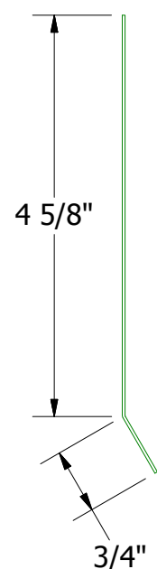
BGA369-Starter Cleat
