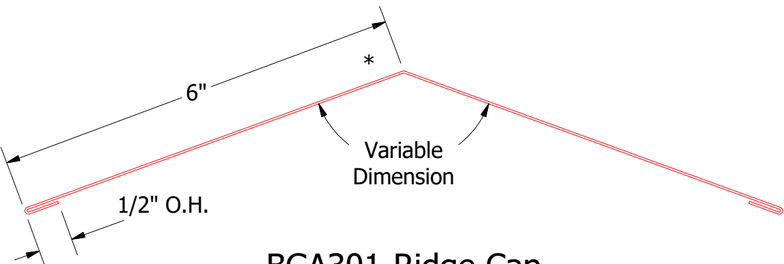
BGA301-Ridge Cap
