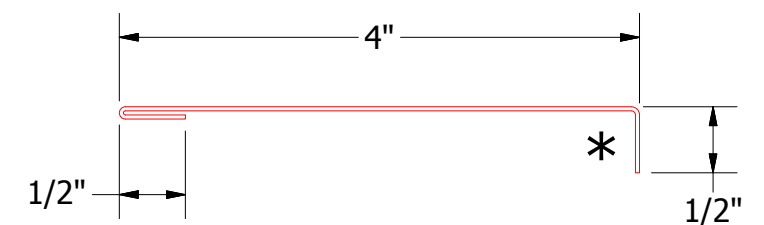
MFA671-Jamb Trim
