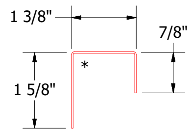
MPA270-J Closure
