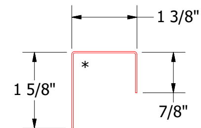
MPA270-J Closure
