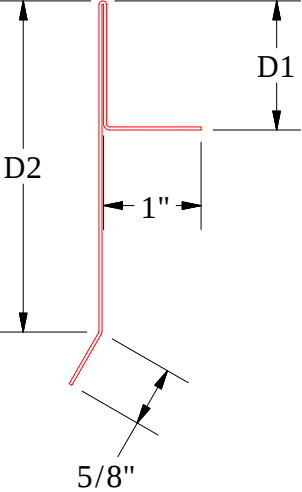
Gable Starter Cleat PCA211 - 1" Seam and 1" Batten D1=1 5/16" / D2=3 7/16" PCA214 - 2" Batten D1=2 5/16" / D2=4 7/16"
