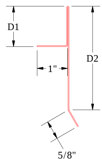
Gable Starter Cleat PCA211 - 1" Seam and 1" Batten D1=1 5/16" / D2=3 7/16" PCA214 - 2" Batten D1=2 5/16" / D2=4 7/16"
