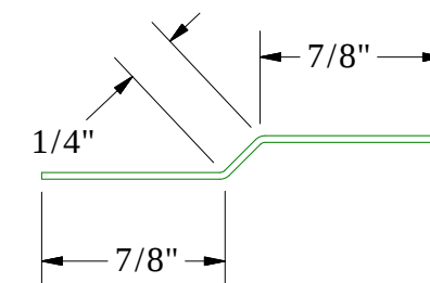
PCA975-Joggle Cleat
