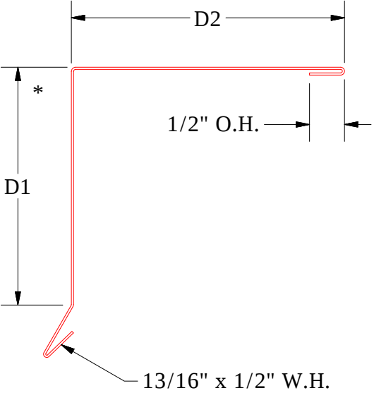
Gable Trim Cap PCA210 - 1" Seam and 1" Batten D1=3 1/2" / D2=4" PCA212 - 2" Batten D1=4 1/2" / D2=5 1/2"
