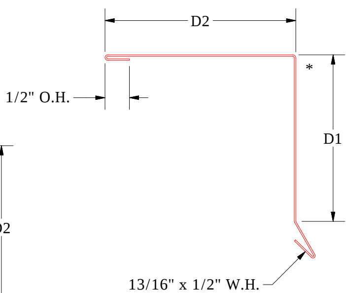
Gable Trim Cap PCA210 - 1" Seam and 1" Batten D1=3 1/2" / D2=4" PCA212 - 2" Batten D1=4 1/2" / D2=5 1/2"
