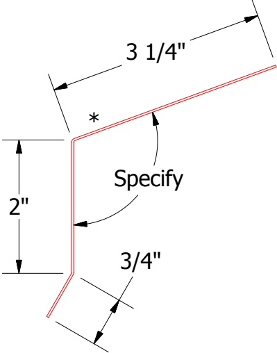
SCA175-Drip Edge
