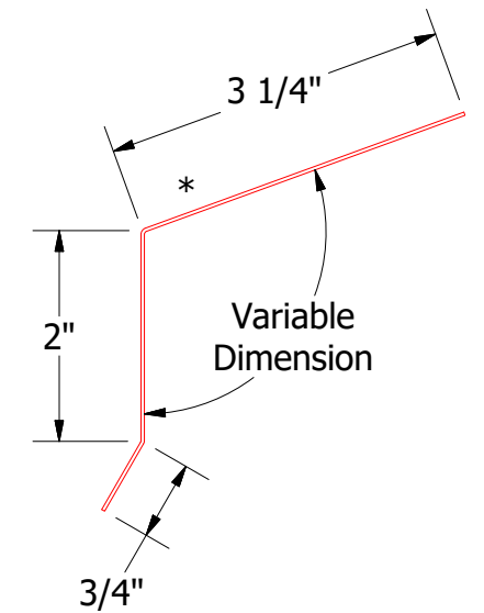
SCA175-Drip Edge
