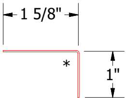
VSA680 - Angle Trim
