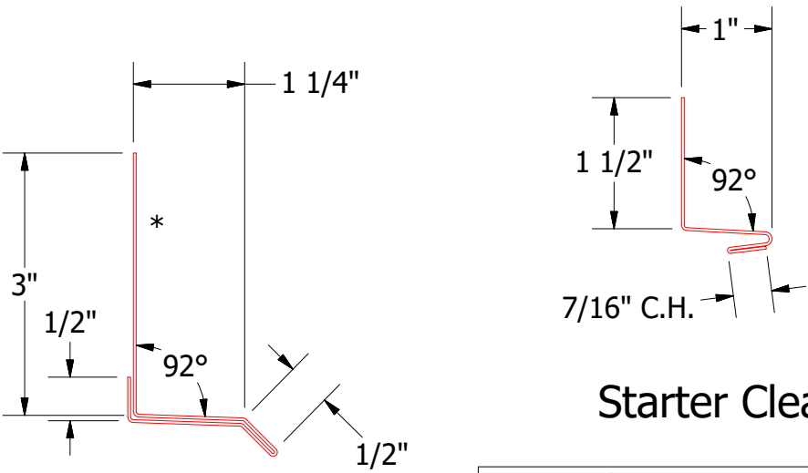
VSA661 - Base Trim
