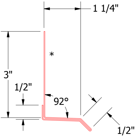
VSA661 - Base Trim
