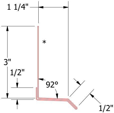
VSA661-Base Trim
