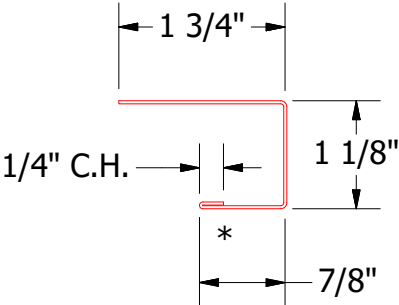
VSA118-J Channel
