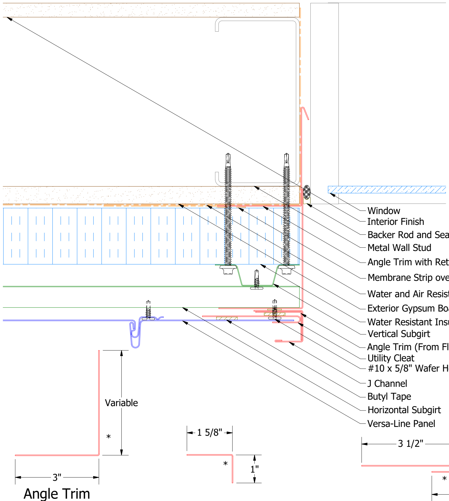
VSA680-Angle Trim
