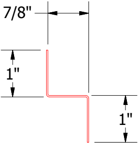
VSA681-Support Z
