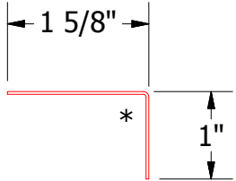
VSA680-Angle Trim
