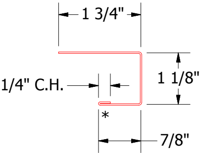
VSA118-J Channel
