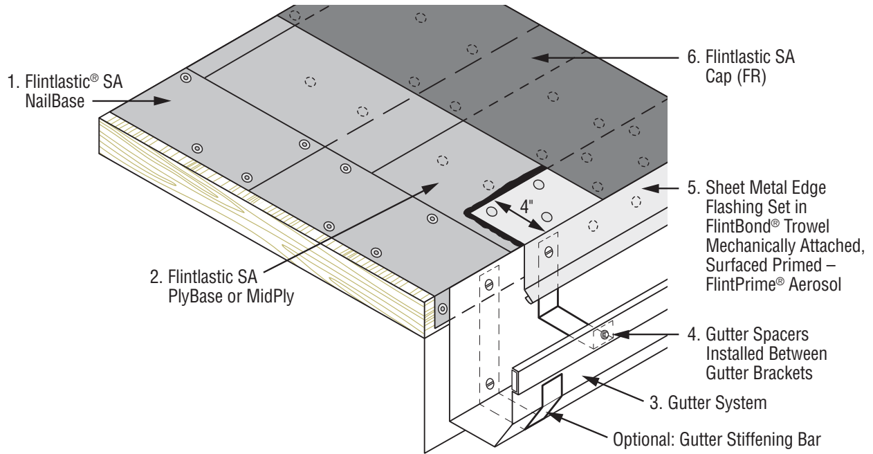
CT-01B Edge Flashing – Gutter
