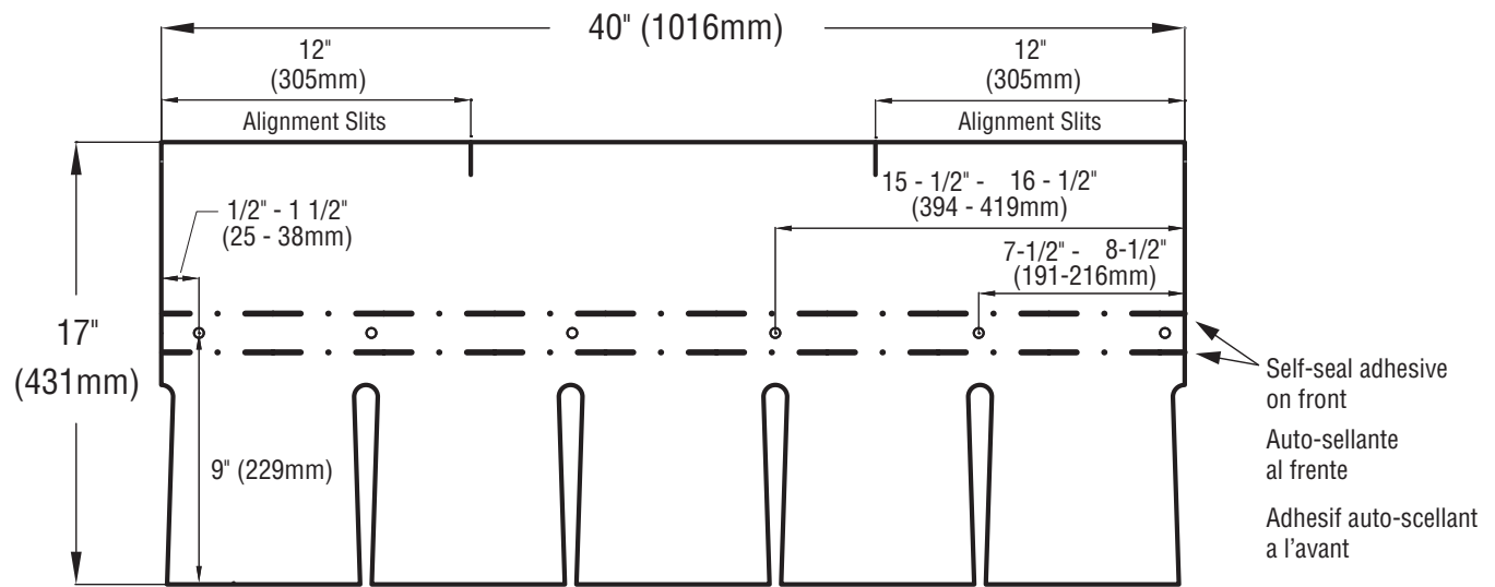
STANDARD NAILING PATTERN - six nails per shingle ESQUEMA DE CLAVADURA ESTÁNDAR - seis clavos por teja PATRON DE CLOUAGE STANDARD - six clous par bardeau
