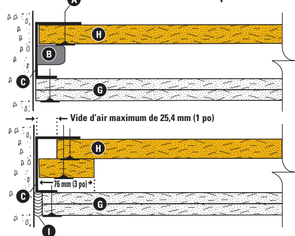
Vue de l'extrémité de la paroi
