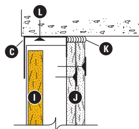
Vue du sommet du mur
