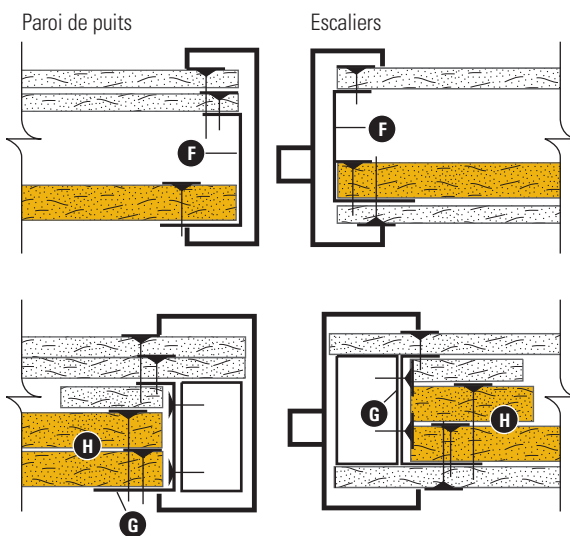
Montant de porte, standard
