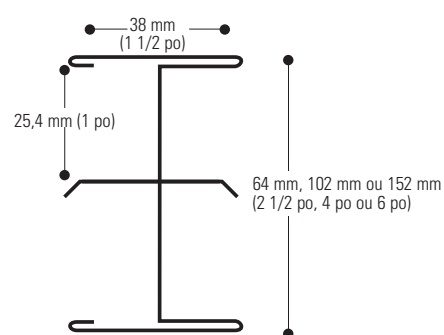
Détail du poteau I
