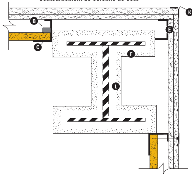
Contournement de colonne de coin
