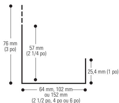
Rail en J
