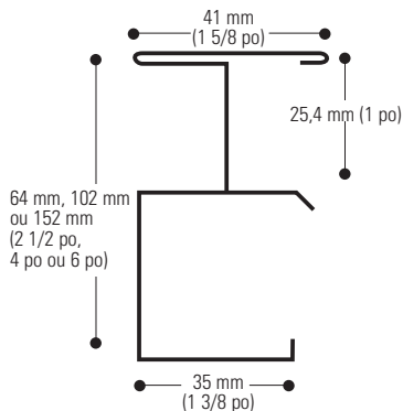
Rail en J
