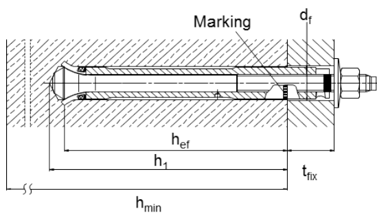
HDA-T / HDA-TR
