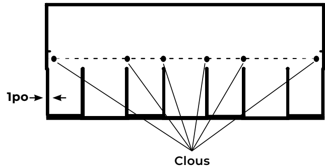
Pente Raide/Grand Vents Nécessite 6 Clous
