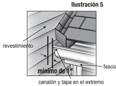
Ilustración 5 Mantenga un espacio mínimo de 1" entre las tapas de los extremos de los canalones y el revestimiento y la moldura.
