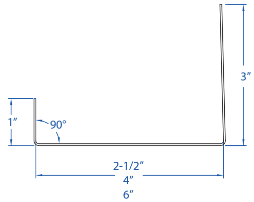
Jamb Track
