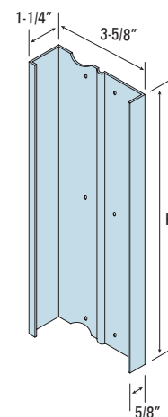
Web Stiffener
