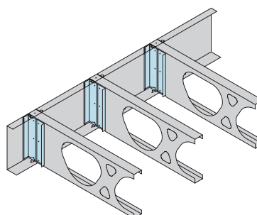
Web Stiffener
