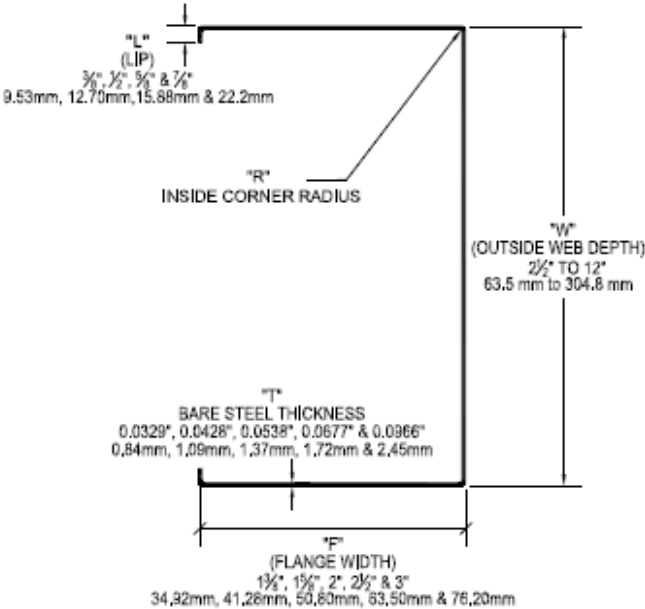
STRUCTURAL STUD
