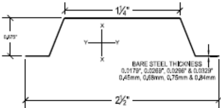
FURRING HAT CHANNEL
