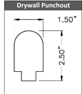
Drywall Punchout
