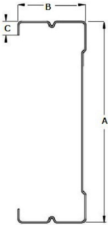
VIPERSTUD
