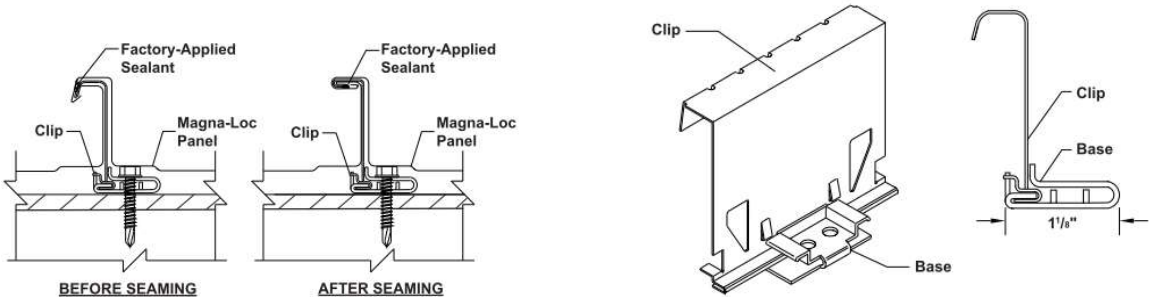
FIGURE 1B—MAGNA-LOC CLIP
