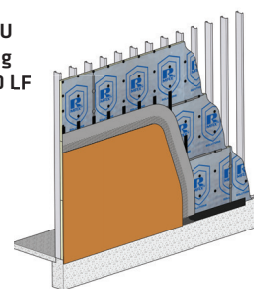
Metal Stud Stucco Cladding R-SEAL 2000 LF
