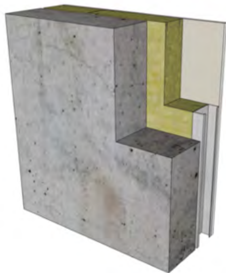
Ensamble de muro de concreto expuesto con aislante en el interior pero sin barrera de vapor de lámina de polietileno en el interior. Este tipo de ensamble puede tener un desempeño durable en climas cálidos.
