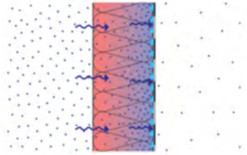
Corte transversal vertical esquemático que muestra la condensación de humedad en un material retardante de vapor colocado en el lado equivocado de un ensamble de muro.
