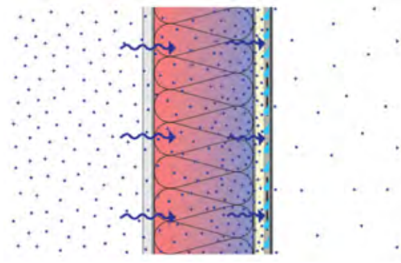
Corte transversal vertical esquemático de un muro con recubrimiento no ventilado impermeable al vapor localizado en un clima frío.
