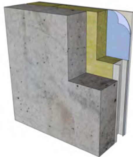
Ensamble de muro de concreto expuesto aislado en el interior como se haría normalmente para clima frío.
