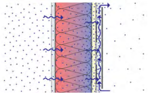
Corte transversal vertical esquemático de muro con recubrimiento impermeable al vapor localizado en un clima frío con ventilación detrás del recubrimiento para permitir la disipación de humedad.
