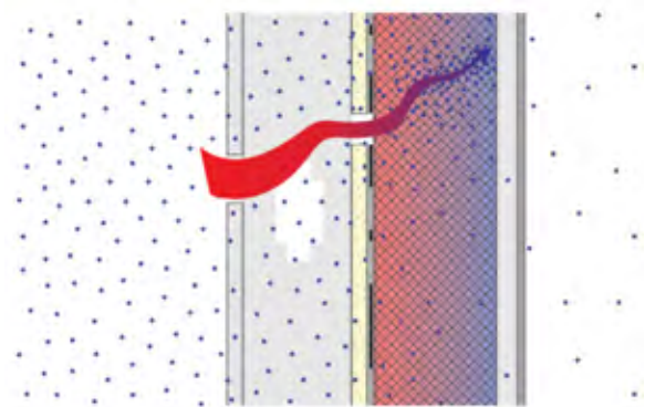
Corte transversal esquemático de un muro aislado en el exterior en un clima frío sin barrera de vapor y filtración de aire.
