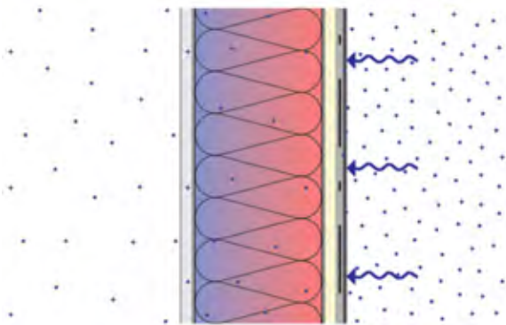
Corte transversal vertical esquemático de muro con control de vapor exterior en un clima cálido que evita que se acumule humedad dentro del ensamble de muro.
