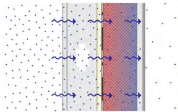
Corte transversal vertical esquemático de un muro aislado en el exterior en un clima frío sin barrera de vapor.
