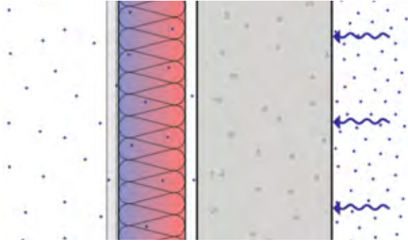
Ensamble de muro de concreto expuesto aislado en el interior pero sin lámina de polietileno como barrera de vapor en el interior. Este tipo de ensamble puede tener un desempeño durable en climas cálidos.
