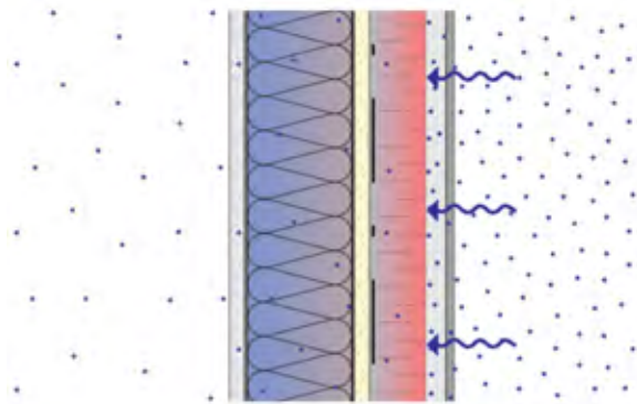
Corte transversal vertical esquemático de un muro con aislante dividido localizado en un clima cálido con aislante exterior impermeable.
