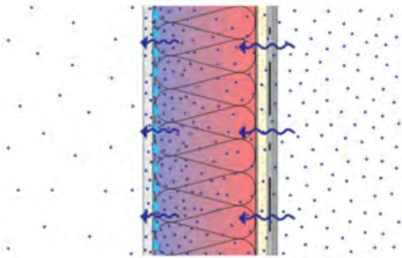
Corte transversal vertical esquemático de muro sin control de vapor exterior en un clima cálido que da como resultado condensación en la cara exterior del revestimiento de yeso interior.
