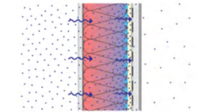
Corte transversal vertical esquemático del muro con membrana de barrera de vapor en el revestimiento del muro exterior en un clima frío.
