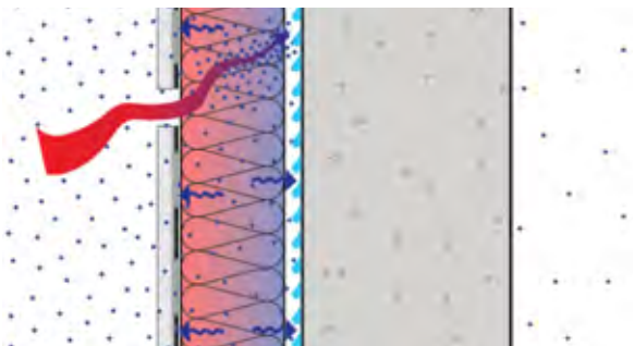
Corte transversal vertical esquemático de un muro de concreto expuesto aislado en el interior con una barrera de vapor interior que muestra cómo la filtración de vapor puede causar acumulación de humedad dentro del ensamble, que no puede secarse debido a las barreras de vapor dobles.
