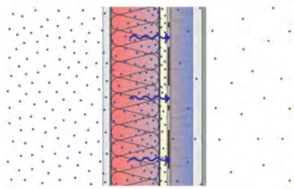
Corte transversal vertical esquemático de un muro con aislamiento dividido localizado en un clima frío con aislamiento exterior impermeable.
