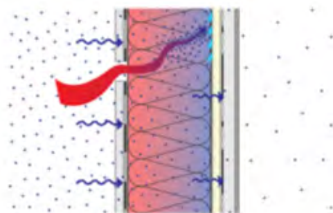
Corte transversal vertical esquemático de un muro que presenta condensación de aire en la cara interior de un revestimiento exterior de yeso.
