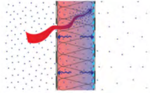
Corte transversal vertical esquemático que muestra la humedad atrapada en un ensamble de muro debido a la presencia de dos barreras de vapor.
