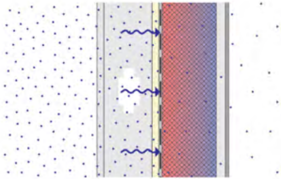
Corte transversal vertical esquemático de un muro aislado en el exterior con membrana de barrera de vapor sobre el revestimiento del muro exterior en un clima frío.
