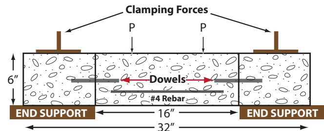
Modified AASHTO T253 Test Diagram
