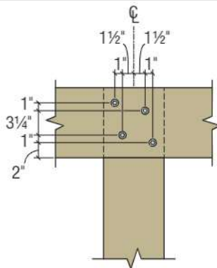
Detail SQ1
