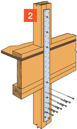
No Sheathing / Sin Relleno
