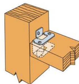
RTRZ Installation
