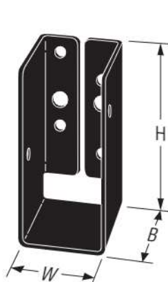
APLH (APHH similar)
