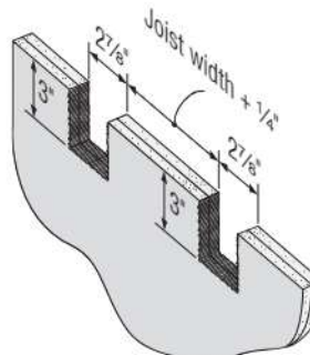
Drywall Notches
