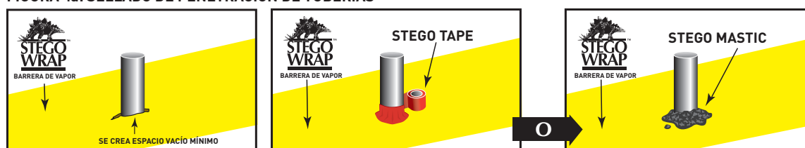
FIGURA 4a: SELLADO DE PENETRACIÓN DE TUBERÍAS
