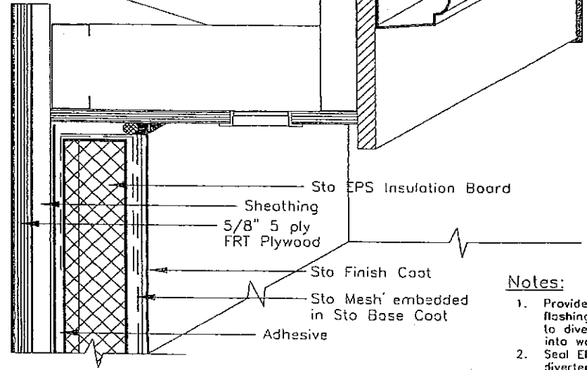
OVERHANG N.T.S.
