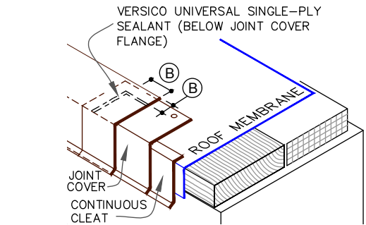
TPC-1.1 VersiTrim Drip Edge Fascia
