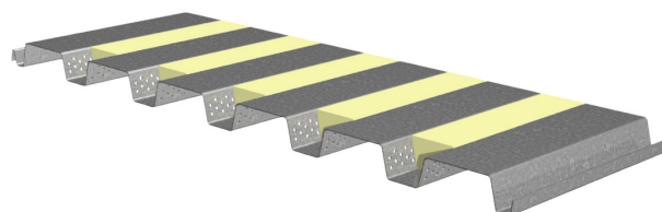
1.5BA-36 / 1.5BIA-36 / 1.5PLBA-36
