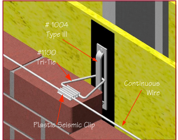
Type III Seismic
