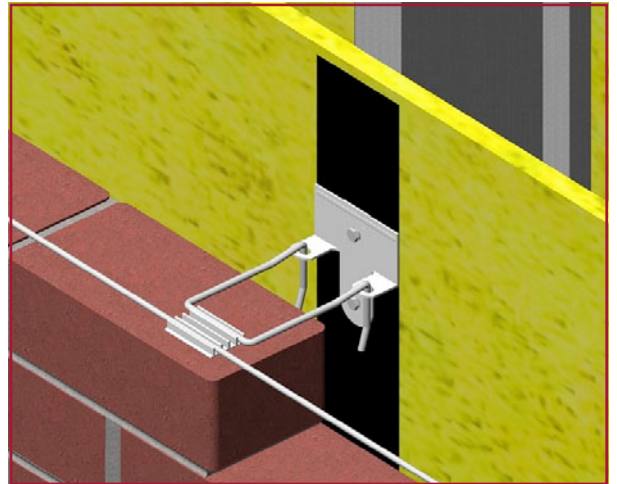
RJ-711 Seismic
